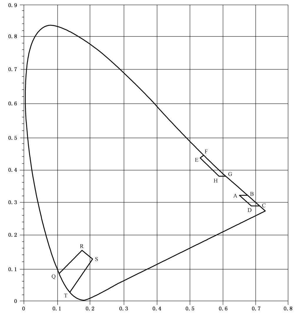
图 A.1 标志灯具灯光颜色色品图
